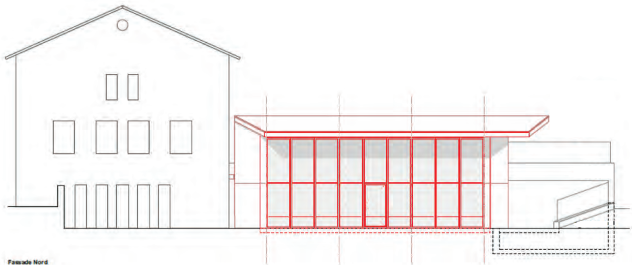
Fassade Nord
